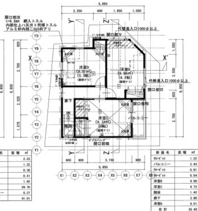
3階平面図 S:1/100
