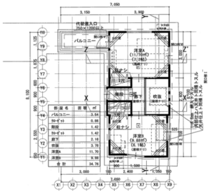
3階平面図 S:1/100
